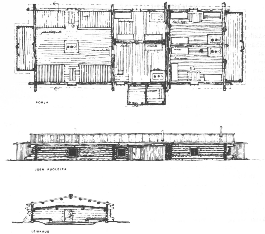
Kuva 3. Pääpirtti, metsähallitus 1933–1936. Mittakaava 1:200. Lähde: JUNTILA ym., 1972.
