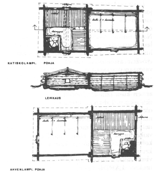
Kuva 2. Kemi Oy:n kämppiä vuosina 1906–1907. Lähde: JUNTILA ym., 1972.
